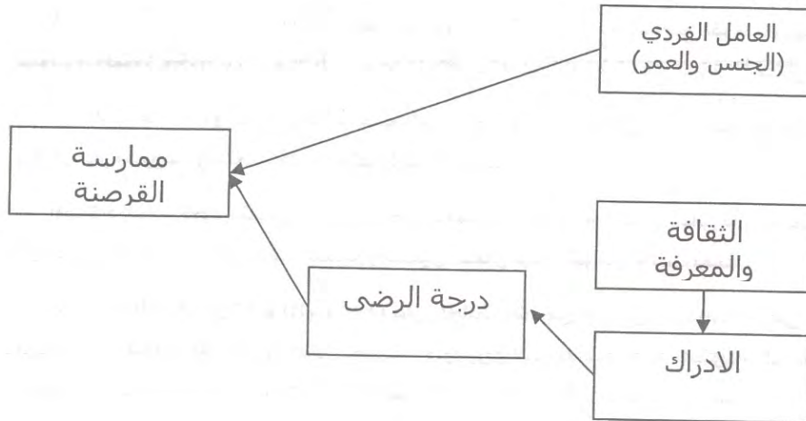
شكل ٢ : نموذج البحث
